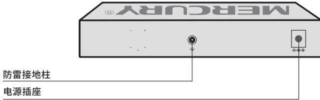
图 2-5 SE106P Pro 后面板示意图
