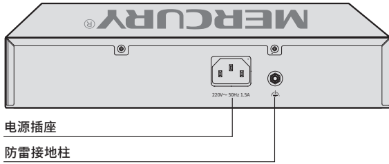
图 2-4 SE109P Pro 后面板示意图
